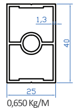
K2208 25x40 Dikme
