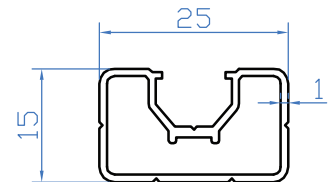
K2356 25x15 DEKO KUTU 0.250 Kg/m
