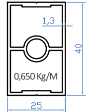
K2208 25x40 Dikme Profil
