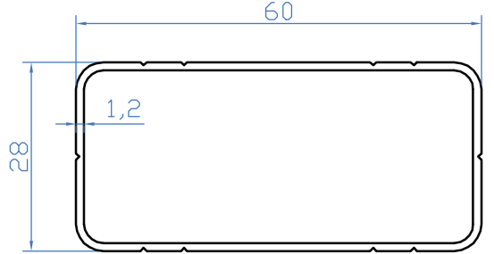
K2300 60x28 DEKO KUTU 0.540 Kg/m
