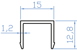
K2304 20x28 DEKO KAPAK 0.125 Kg/m
